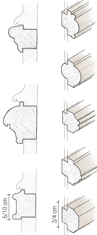
Traverses d'impostes
