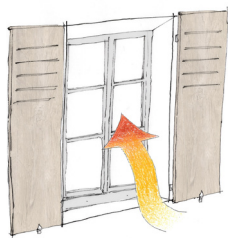
Apports solaires (chaleur, lumière) et ventilation naturelle
